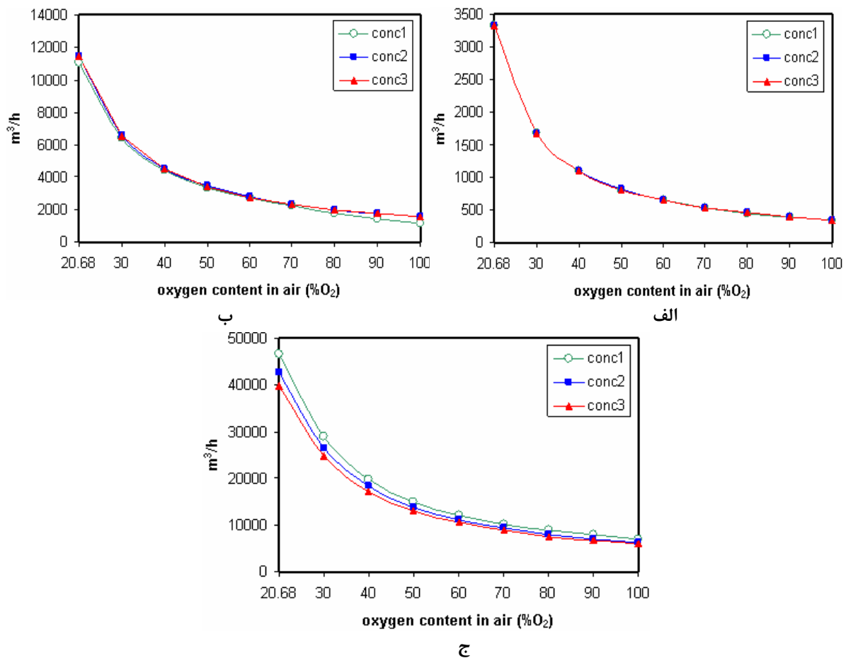
شکل 5- تأثیر نوع کنسانتره بر مقدار هوای مصرفی در (الف) ستلر (ب) آپتیک (ج) محفظه واکنش.
