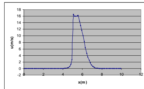
شکل ۱۸: پروفیل سرعت به دست آمده توسط مدل عددی.
