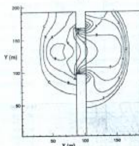
شکل ۱۳: منحنی میزان رقوم سطح آب به دست آمده در مرجع [۳] در آزمون شکست جزئی سد بعد از 7/2 ثانیه.
