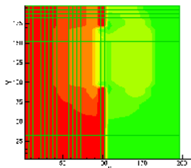
شکل ۱۲: منحنی میزان رقوم سطح آب به دست آمده در مدل حاضر در آزمون شکست جزئی سد بعد از 7/2 ثانیه.
