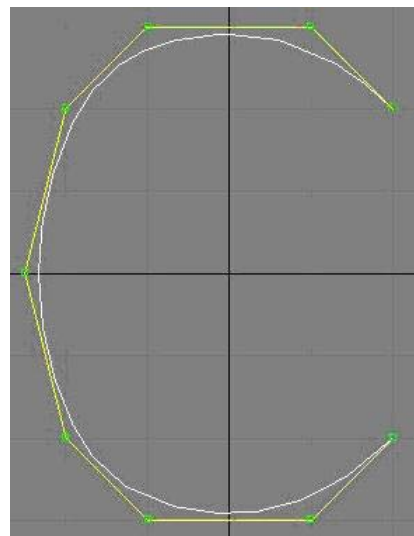
شکل ۵: منحنی NURBS ترسیم شده توسط 3Ds Max
