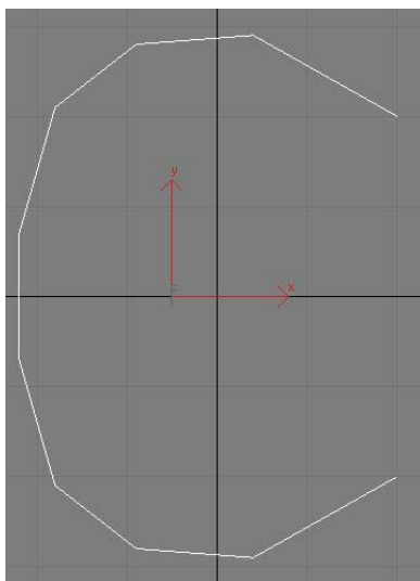
شکل ۶: منحنی NURBS نقاط قبلی با استفاده از کدنویسی رابطه
