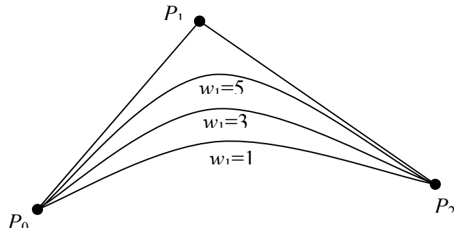
شکل ۳: با افزایش وزن نقاط، منحنی به سمت آن نقطه کشیده می شود
