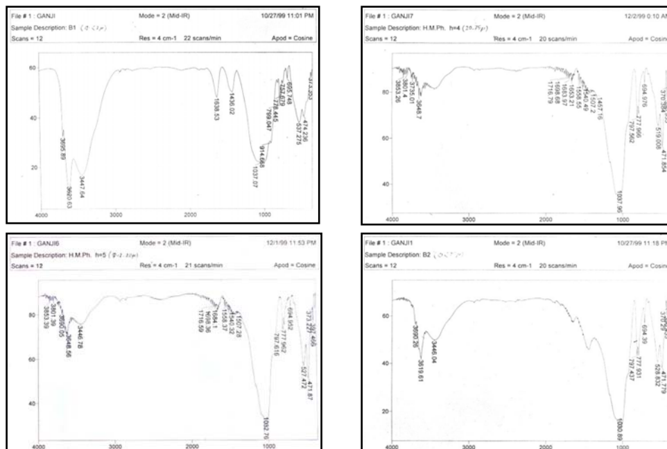
شکل ۳: طیف های جذبی مادون قرمز چهار نمونه از خاک صنعتی بوبین زهرا با قطر دانه های مختلف بالا سمت راست: \Phi=20-75 \mu\text{m} ، پایین سمت راست: \Phi < 75 \mu\text{m} ، بالا سمت چپ: \Phi < 2 \mu\text{m} پایین سمت چپ: \Phi=2-20 \mu\text{m}
