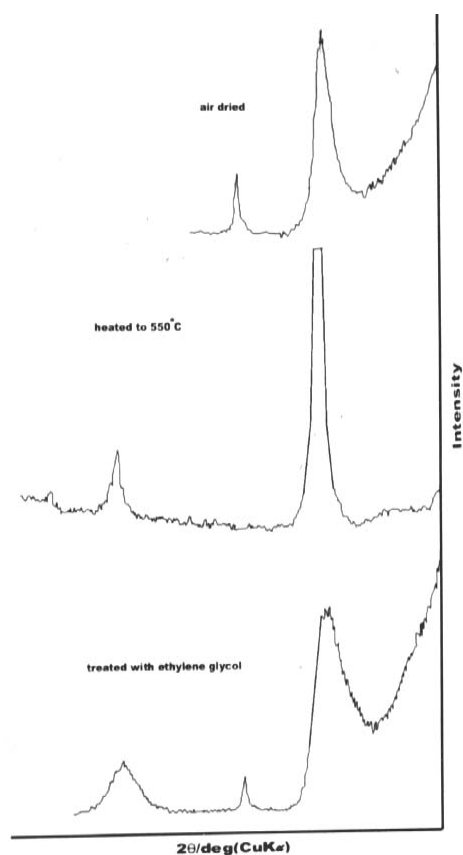
شکل ۲: الگوهای پراش اشعه X نمونه خالص سازی شده (با ابعاد کوچکتر از 2\ \mu\text{m} ) خاک صنعتی بوبین زهرا به ترتیب از بالا به پایین در شرایط؛ خشک شده در هوا، حرارت دیده در دمای 550^\circ\text{C} و عمل آوری شده با اتیلن گلیکول
