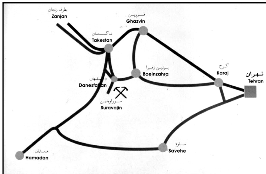
شکل ۱: موقعیت و راههای دسترسی معدن خاک صنعتی بویین زهرا
