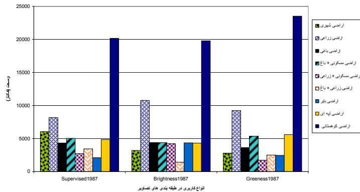
شکل ۲ - انواع کاربری اراضی در طبقه بندی های تصاویر سال ۱۹۸۷
