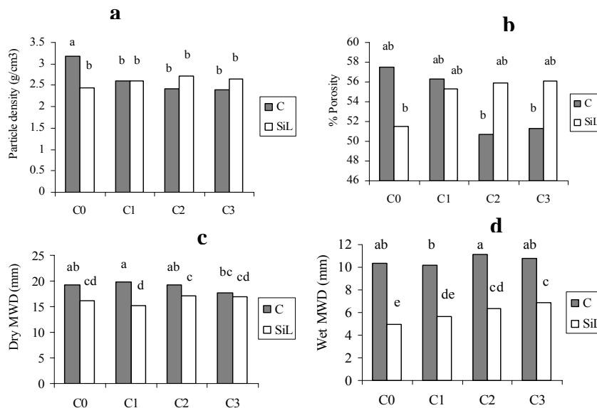
شکل ۴- مقایسه میانگین اثر متقابل خاک و سطح اختلاط بر جرم مخصوص حقیقی (a)، تخلخل (b)، خشک (c) و MWD خیس (d)، [C خاک رسی، SiL خاک لوم سیلتی، C0 سطح اختلاط صفر، C1 (۷۵ متر مکعب در هکتار)، C2 (۱۵۰ متر مکعب در هکتار) و C3 (۳۰۰ متر مکعب در هکتار)]
