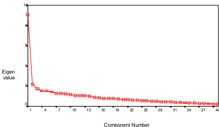
نمودار ۱. نمودار اسکری برای نشان دادن عامل‌های مشترک
