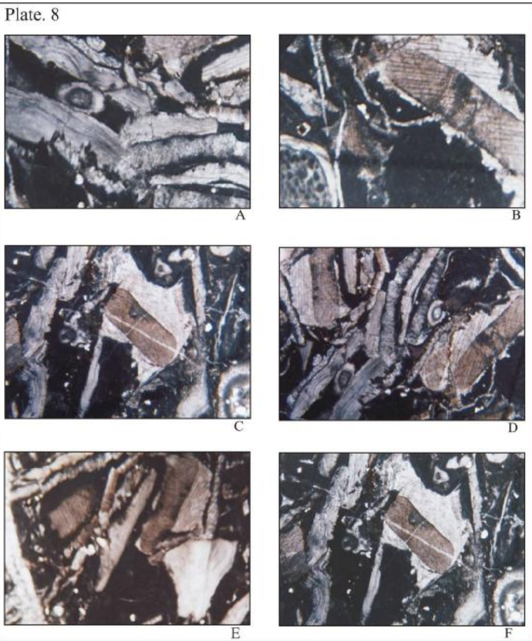
A, D - براکیوپود پکستون ۲۰ × وجود فونای دریای باز از قبیل براکیوپود حاکی از تشکیل رخساره مزبور در بخش جلویی سد بیوکلاستیک است.
