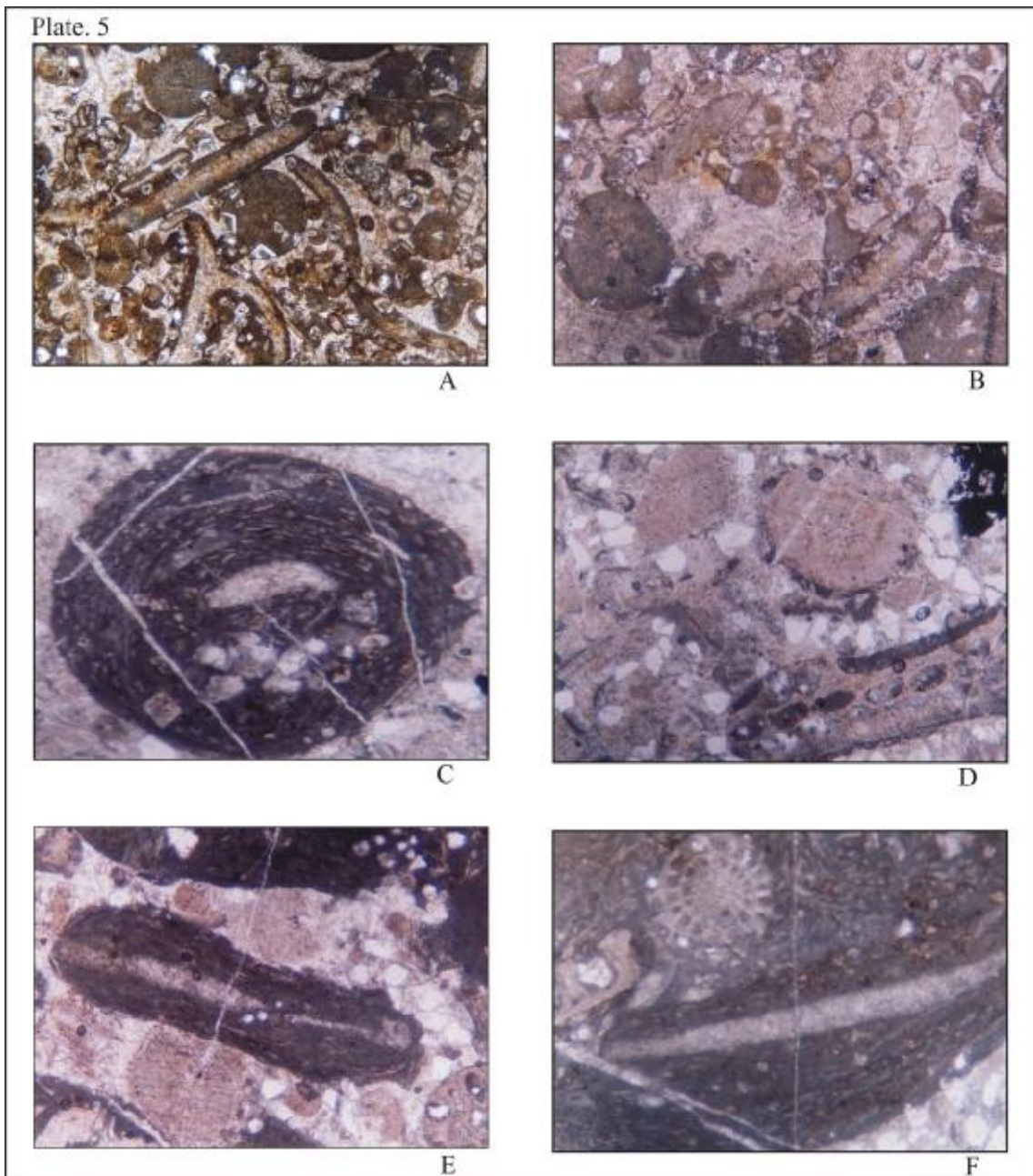
A, B - بیوکلاست اووئید گرینستون ۲۰ ×
