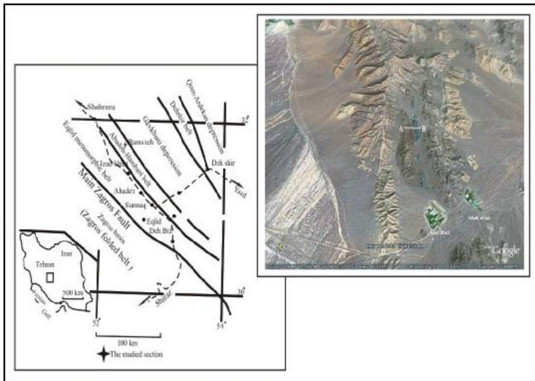
شکل ۲: زون های ساختاری منطقه شهرضا - ده بید - آباد (گروه ایرانی ژاپنی، ۱۹۸۱) - تصویر ماهواره ای مقطع مورد مطالعه.
