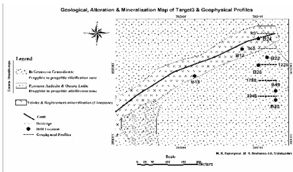
نقشه ۸- موقعیت پروفیل‌های مغناطیسی منطقه اکتشافی (۳) بر روی نقشه زمین‌شناسی - آلتراسیون - کانی‌سازی
