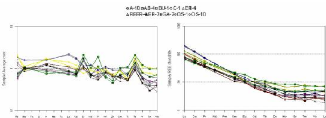
تصویر ۲۳: بهنجار سازی نمونه ها با کندریت تصویر ۲۴: بهنجار سازی نمونه ها با میانگین پوسته
