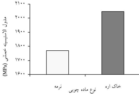
شکل 5- تاثیر مستقل نوع ماده چوبی بر مدول الاستیسیته خمشی
