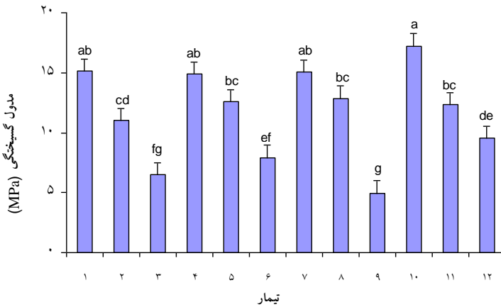
شکل 1- مقایسه و دسته‌بندی میانگین‌های مدول گسیختگی 12 تیمار.
