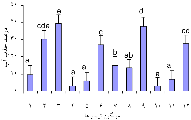
شکل 9- مقایسه و دسته‌بندی میانگین‌های درصد جذب آب بعد از 2 ساعت
