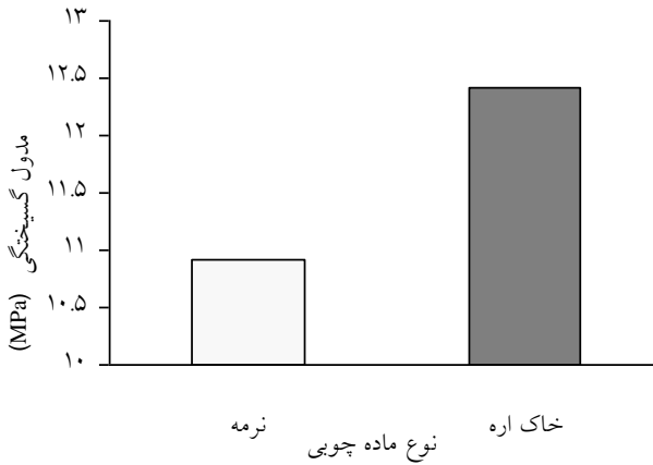
شکل 2- تاثیر مستقل نوع ماده چوبی بر مدول گسیختگی
