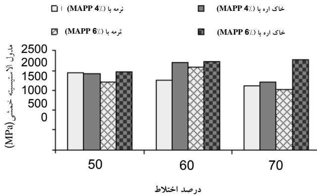
شکل 6- تاثیر متقابل ماده چوبی، درصد اختلاط و MAPP بر مدول الاستیسیته خمشی
