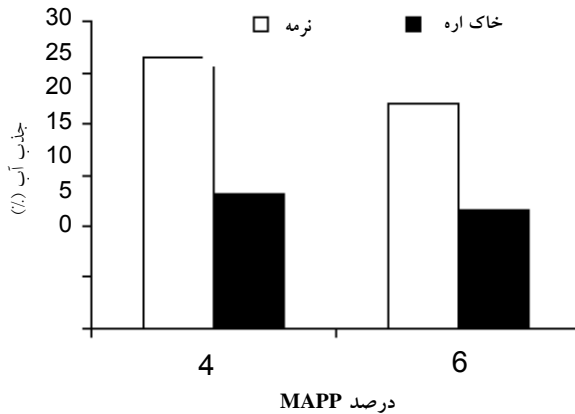
شکل 10- تاثیر متقابل ماده چوبی و MAPP بر درصد جذب آب 2 ساعت
