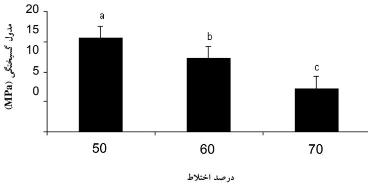
شکل 3- تاثیر مستقل درصد اختلاط بر مدول گسیختگی
