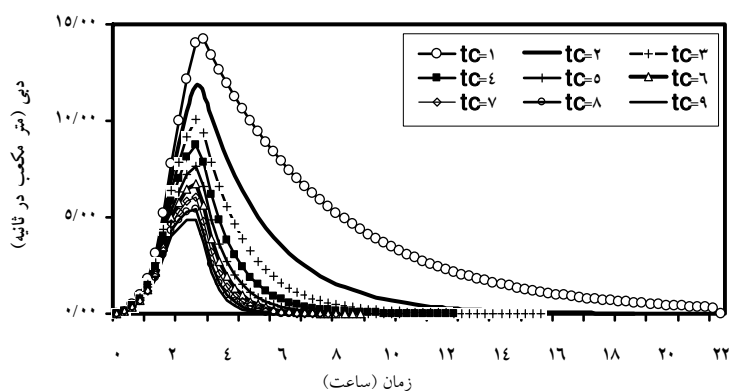
شکل ۶- نتایج آنالیز حساسیت مدل هیدروگراف واحد لحظه‌ای کلارک برای مقادیر متفاوت زمان تمرکز (ساعت).
