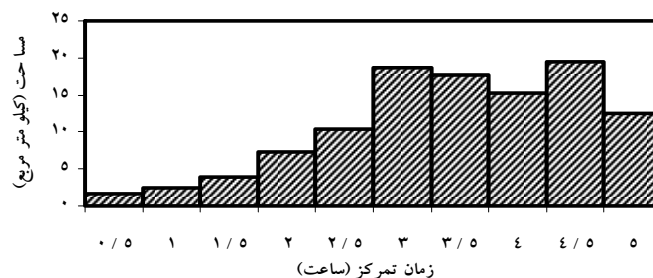
شکل ۳- هیستوگرام زمان مساحت آبخیز جعفرآباد.
