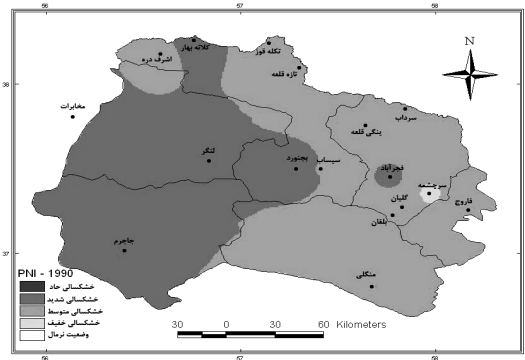
شکل ۱- پهنه‌بندی خشک‌سالی هوشناسی با استفاده از SPI (الف)، DI (ب) و PNI (ج) در استان خراسان شمالی در سال ۱۹۹۰.
