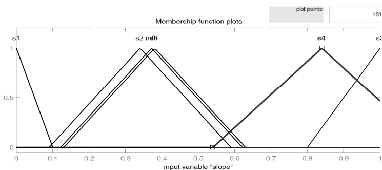
شکل ۲- تابع عضویت مثلثی عامل درصد شیب.
