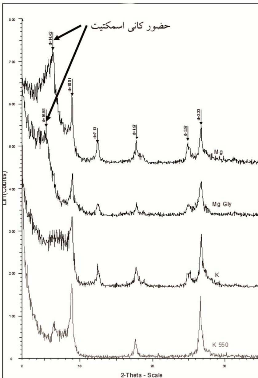
شکل ۳- پرتونگراشعه ایکس بخش رس، پیک 17\text{\AA} در تیمار گلیسرول نشان‌دهنده کانی اسمکتیت می‌باشد (سری خاک قره‌سو، افق A_p ).
