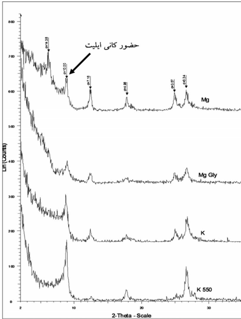
شکل ۲- پرتونگار اشعه ایکس بخش رس، پیک 10^{\circ}A نشان دهنده کانی ایلیت می باشد (سری خاک مینودشت، افق B_{k1} ).
