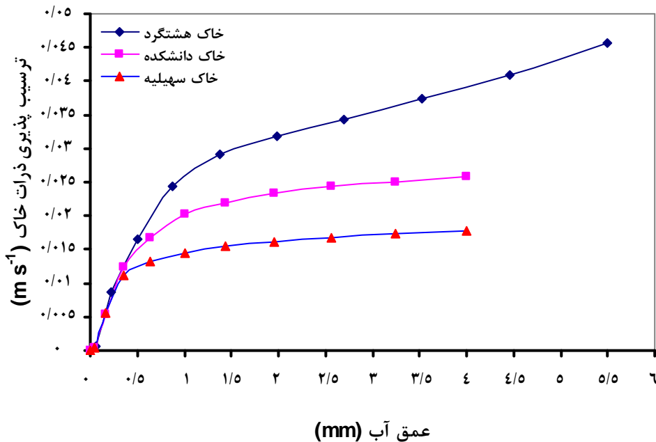
شکل ۲- مقادیر ترسیب پذیری ذرات خاک ( \theta ) در عمق‌های مختلف آب برای سه خاک مورد مطالعه.
