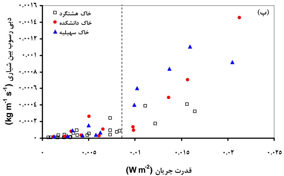
شکل ۱- تغییرات دبی رسوب با افزایش قدرت جریان رواناب حاصل از باران شبیه‌سازی شده برای (الف) میانگین داده‌ها در شرایط پایدار و (ب) میانگین کل رخداد بارش در سه خاک مورد مطالعه.
