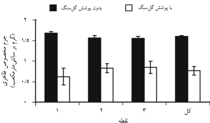
شکل ۵- نمودار مقایسه میانگین جرم مخصوص ظاهری در خاک‌های دارای پوشش گل سنگ و بدون پوشش گل سنگ.
