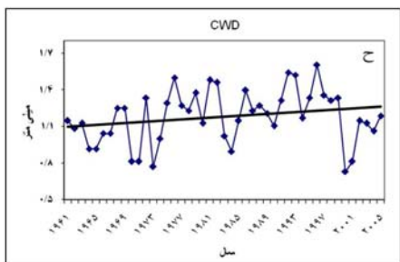
شکل ۲- سری زمانی فراوانی‌های بارش بر اساس صدک‌های آستانه، حداکثر شدت بارش یک روزه، طول روزهای پیوسته خشک و مرطوب برای دوره ۱۹۶۱-۲۰۰۵.
