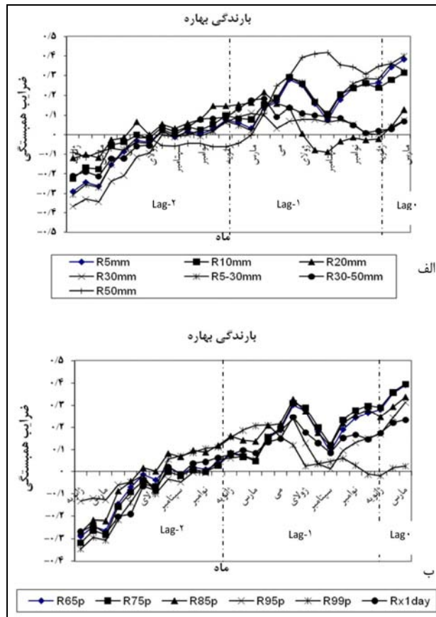
شکل ۴- همبستگی مقادیر حدی بارش بهار و دمای سطح اقیانوس در ناحیه نینو ۳.۴ در سه وقفه زمانی مختلف در استان خراسان بزرگ.
