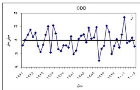
شکل ۲- سری زمانی فراوانی‌های بارش بر اساس صدک‌های آستانه، حداکثر شدت بارش یک روزه، طول روزهای پیوسته خشک و مرطوب برای دوره ۱۹۶۱-۲۰۰۵.
