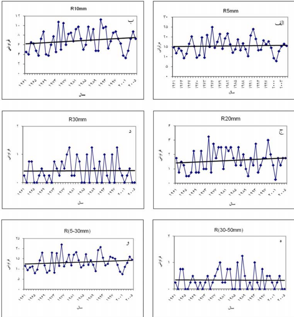
شکل ۱- سری زمانی فراوانی‌های بارش بر اساس آستانه‌های ثابت برای دوره ۱۹۶۱-۲۰۰۵.
