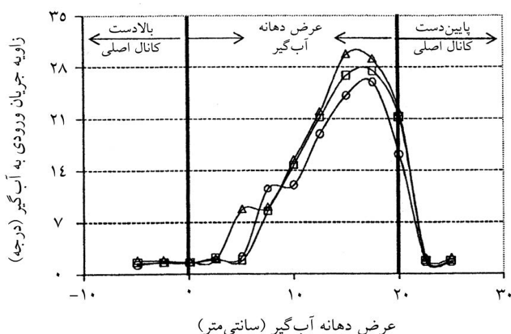
شکل ۲- زاویه بردار سرعت در مقابل دهانه آب‌گیر در لایه نزدیک کف.
