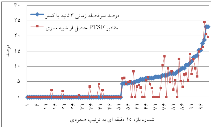
نمودار شش: مقایسه درصد سرفاصله زمانی و PTFSF در بازه ۱۵ دقیقه‌ای، راه دوخطه زنجان-میانه
