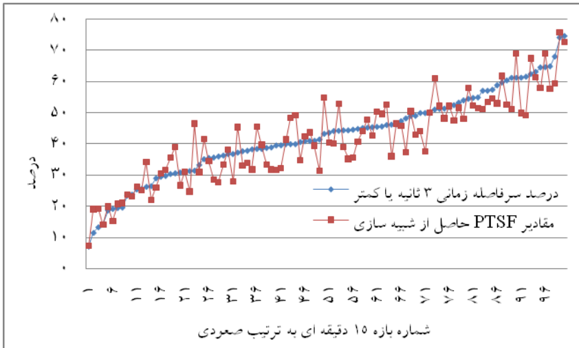
نمودار پنج: مقایسه درصد سرفاصله زمانی و PTFSF در بازه ۱۵ دقیقه‌ای، راه دوخطه کرج-چالوس
