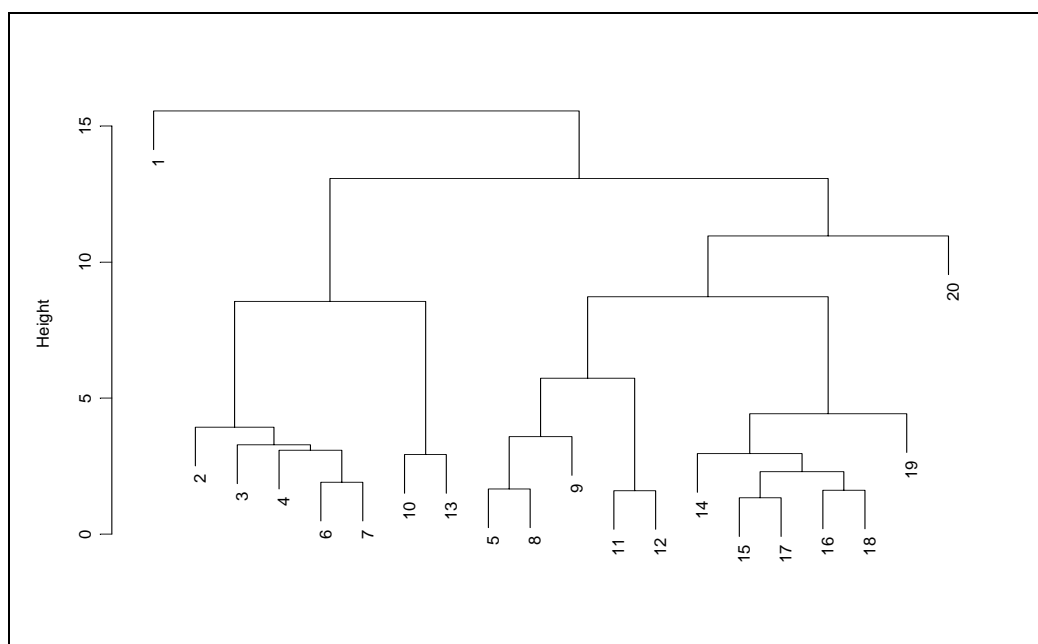
شکل ۳- نمودار داربستی تفکیک حوضه ها بر اساس مشابهت متغیرهای ژئومورفیک موثر بر سیلاب زیر حوضه‌ها
