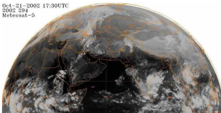
شکل ۳۹- تصویر ماهواره ای مادون قرمز Meteosat5 در تاریخ ۲۱ اکتبر ۲۰۰۲ و ساعت ۱۸. در این
