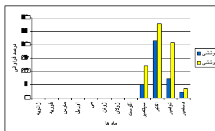
شکل ۱۸- رژیم ماهانه فراوانی ابرهای پوششی و جوئشی در زمان وقوع رویدادهای بارشی فوق سنگین ایستگاه بابلسر
