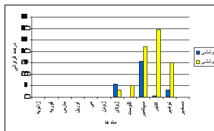
شکل ۲۰- رژیم ماهانه فراوانی ابرهای پوششی و جوئشی در زمان وقوع رویدادهای بارشی فوق سنگین ایستگاه آستارا
