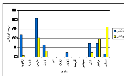
شکل ۱۴- رژیم ماهانه فراوانی ابرهای پوششی و جوئشی در زمان وقوع رویدادهای بارشی فوق سنگین ایستگاه
