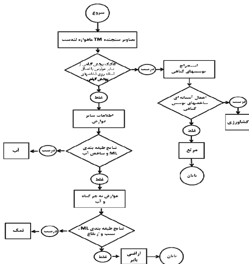
شکل ۵- مدل طراحی شده مبتنی بر خوارزمیک درخت تصمیم برای استخراج نقشه کاربری اراضی در این تحقیق
