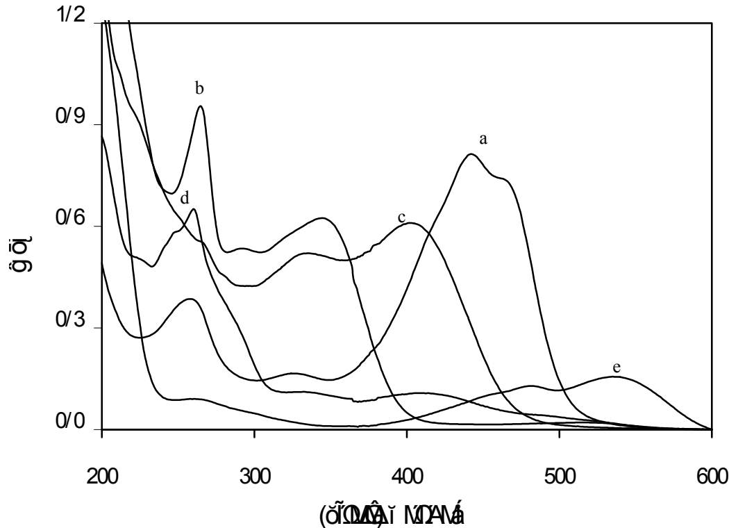
شکل ۱: طیف‌های فرابنفش- مرئی حلول آبی- متانولی (۵۰٪ حجمی/ حجمی) زعفران خالص (۰/۰۱ میلی گرم بر میلی لیتر a) و خامه‌های رنگ شده با رنگهای استخراج شده از گلبرگ زعفران (۰/۲۵ میلی گرم بر میلی لیتر b)، گلرنگ (۰/۱۵ میلی گرم بر میلی لیتر c)، روناس (۰/۱۷ میلی گرم بر میلی لیتر d) و چغندر قرمز (۲ میلی گرم بر میلی لیتر e).
