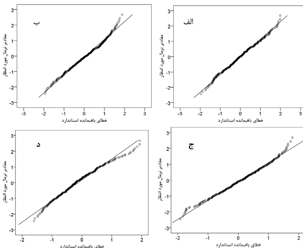
شکل ۴- نمودارهای احتمال نرمال خطای باقیمانده مدل‌ها، الف: جذر سطح مقطع و باندهای اصلی، ب: لگاریتم سطح مقطع و باندهای اصلی و مصنوعی، ج: جذر تعداد در هکتار و باندهای اصلی و د: تعداد در هکتار و باندهای اصلی و مصنوعی
