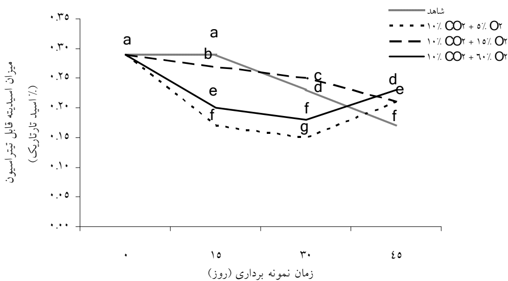
(شکل ۳) - روند تغییرات اسیدیتته قابل تیتراسیون در طی زمان
