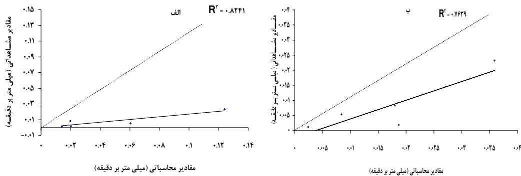
شکل ۷- مقایسه نسبت مقادیر برآورد شده و مقادیر واقعی هدایت هیدرولیکی عمودی خاک با بافت رسی برای الف) مدل رگرسیونی و ب) مدل عصبی- فازی. خط ممتد بیانگر خط رگرسیونی و خط منقطع بیانگر خط ۱:۱ می‌باشد.
