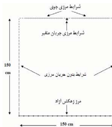
شکل ۱- پروفیل شبیه‌سازی شده و شرایط اعمال شده در مدل HYDRUS-2D
