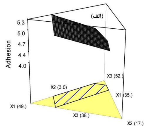
شکل ۱۲: (الف) سطح پاسخ و (ب) تأثیر فاکتورها بر چسبندگی.
