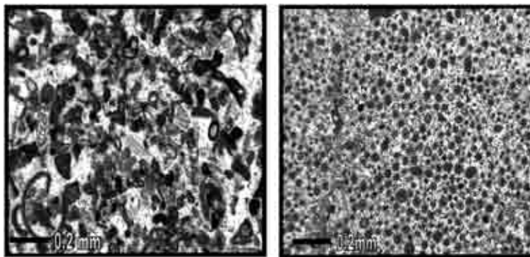
شکل ۹- تصاویر میکروسکوپی از میکروفاسیس پلوئید، اوئید گرینستون دانه ریز واحد دالان بالائی درکوه سورمه (تصویر سمت راست) همراه با تخلخل قالبی و بیوکلاست، پلوئید گرینستون دانه ریز واحد دالان بالائی کوه دنا (تصویر سمت چپ)، ppl.
