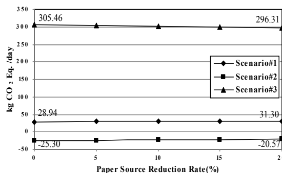
شکل شماره (۴): تجزیه و تحلیل حساسیت سناریوها نسبت به ایجاد کاهش از مبداء تولید دورریزهای کاغذ و مقوا
