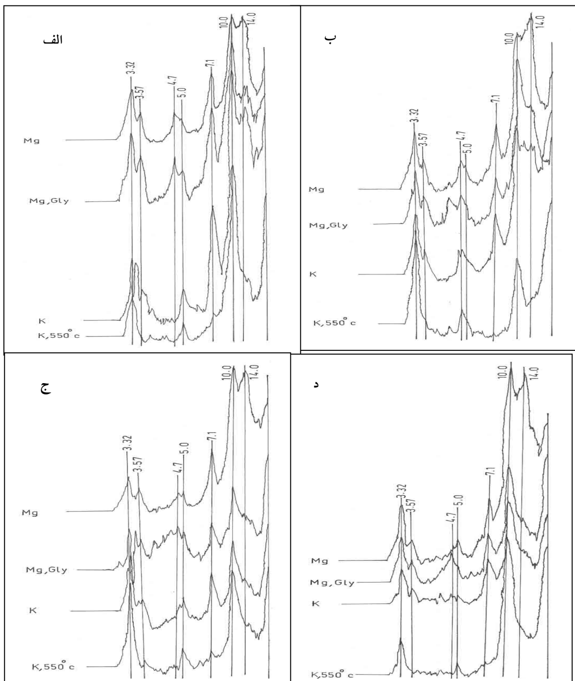
شکل ۲- منحنی‌های اشعه ایکس اف‌های خاک گرگان. الف: پروفیل هموار افق A ۱۵-۰ cm، ب: پروفیل هموار افق Bk ۱ ۸۲-۳۵ cm، ج: پروفیل شانه شیب افق A ۱۶-۰ cm، د: پروفیل پنجه شیب افق Ap ۲۲-۰ cm.
