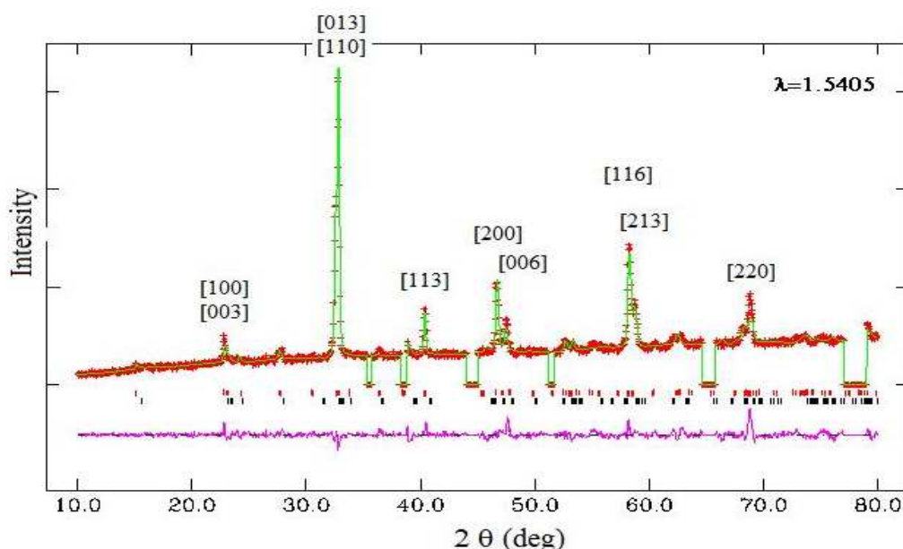
شکل ۱ الگوی پراش برای نمونه بدون جانشینی پتاسیم ( X \approx 0 ). قله‌های ناخالصی حذف شده‌اند (برای توضیح بیشتر به متن مراجعه شود) قله‌های اصلی نمونه نمایه گذاری شده‌اند.
