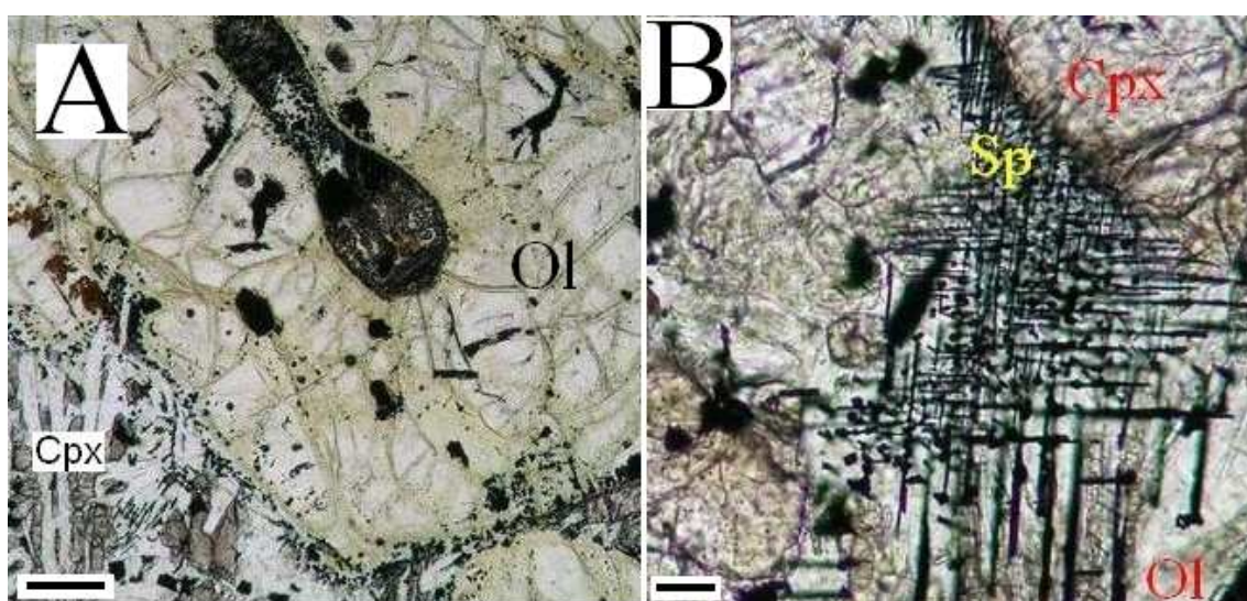
شکل ۷ A مذاب درگیر در بلور الیوین. B تبلور اسپینل‌های متقاطع در فضای بین بلورهای الیوین و کلینوپیروکسن. هر دو تصویر در وضعیت PPL تهیه شده‌اند. مقیاس رسم شده در شکل‌های A و B به ترتیب برابر با ۰/۱۱۵ و ۰/۰۳ میلی‌متر است.
