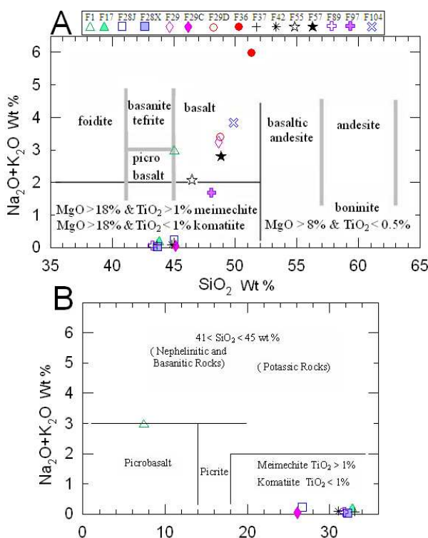
شکل ۲ نام گذاری نمونه‌های فریمان با استفاده از نمودارهای TAS و اکسید منیزیم نسبت به مجموع قلیایی‌ها [۱۵].
