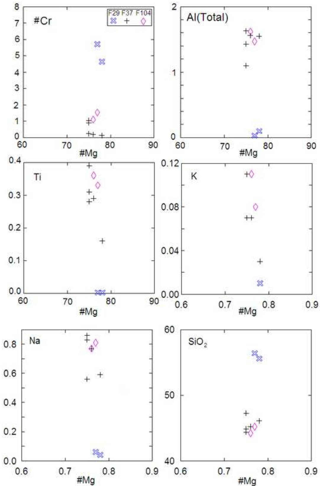
شکل ۱۷ چگونگی تغییرات عدد منیزیم نسبت به عدد کرم، آلومینیم، تیتانیم، پتاسیم، سدیم و سیلیس در ترکیب آمفیبول‌های نمونه‌های الترامافیک F37 (پیکریتی) و نمونه‌های مافیک F104 و F29 (توله ایتی).
