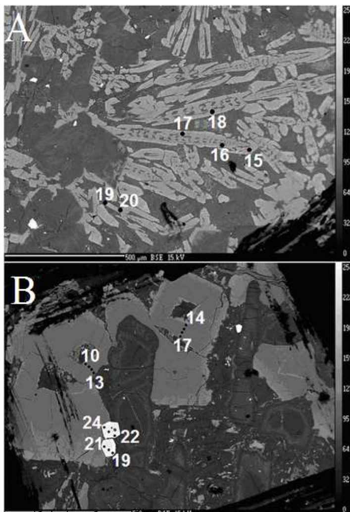
شکل ۵ A تصویر پس پراکندگی (Backscattered Electron Image) نمونه سنگ‌های مافیک پورمعافی، وثوقی عابدینی، امامی و سوزنی را می‌توان ملاحظه کرد. B تصویر نمونه F29C، دو اسپینل خود شکل دیده می‌شوند. شماره‌ها نقاط تجزیه این کانی‌ها را نشان می‌دهند.
