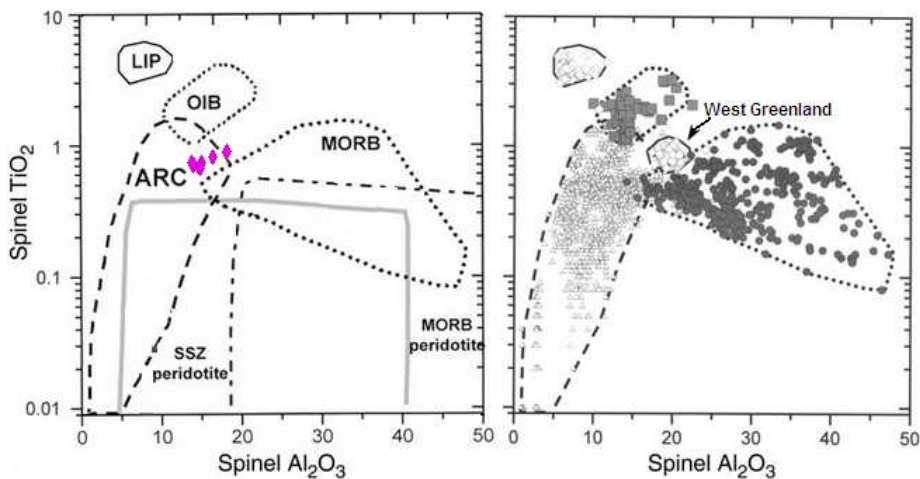
شکل ۱۶ بررسی جایگاه زمین‌ساختی نمونه کوماتی‌ایتی F29C فریمان بر اساس میزان Al_2O_3 و TiO_2 اسپینل‌ها. با مقایسه نمودارهای A و B می‌توان دریافت که اسپینل‌های نمونه کوماتی‌ایتی فریمان مجاور گستره نبود داده‌های مربوط به جایگاه قوسی (ARC) و در همپوشی با گستره مربوط به جایگاه ایالت گسترده آذرین (LIP) غرب گرینلند قرار گرفته‌اند [۳۱].
