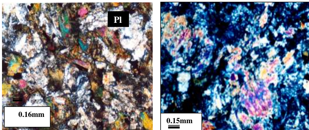
شکل ۵ ب: نمائی از یک گابروی شدیداً رودنژیته شده، XPL. شکل ۵ الف: نمائی از یک گابرو کم رودنژیته شده، XPL
