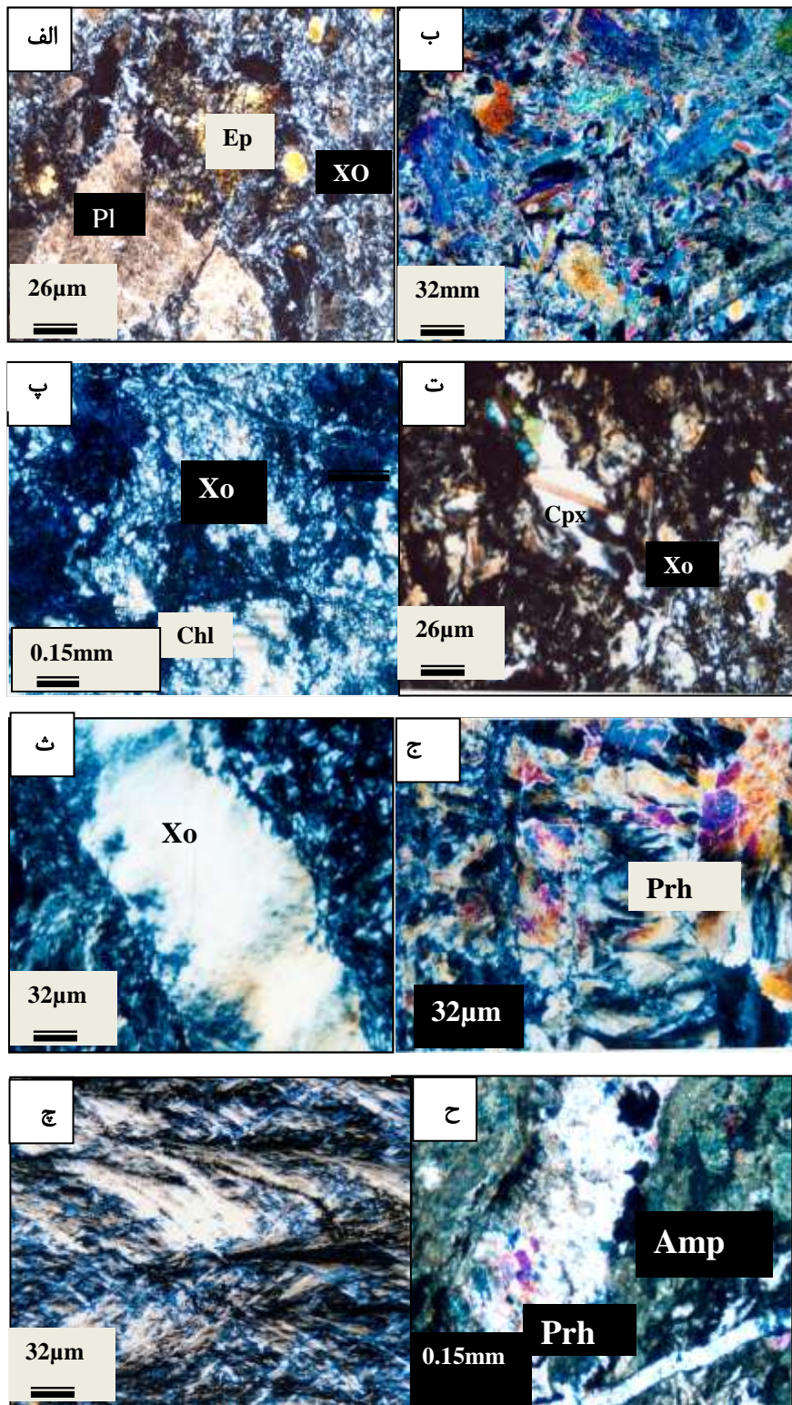
شکل ۶ تصاویر میکروسکوپی رودنژیت‌های افیولیت ملانژ نائین. الف: تبدیل پلاژیوکلاز به اپیدوت در یک گابروی رودنژیته شده ب: تبدیل پلاژیوکلاز به پرنیت در یک گابروی رودنژیته شده پ: تبدیل پیروکسن به کلریت منیزیم‌دار در یک گابروی رودنژیته شده ت: تبدیل پیروکسن-های اولیه به پیروکسن‌های ثانویه در یک گابروی رودنژیته شده ث: زنونلایت رگه‌ای در یک گابروی رودنژیته شده ج: پرنیت رگه‌ای در یک
