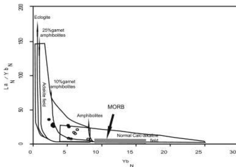
شکل ۱۲ نمودار LaN/YbN نسبت به YbN بهنجار شده با کندریت [۳۱، ۲۱] برای جدایش سنگ‌های آهکی - قلیایی عادی از آداکیت‌ها و موقعیت سنگ‌های مورد بررسی در آن‌ها همراه با منحنی‌های ذوب آمفیبولیت و اکلوزیت و موقعیت متوسط بازالت پشته‌ی میان اقیانوسی [۱۸]
