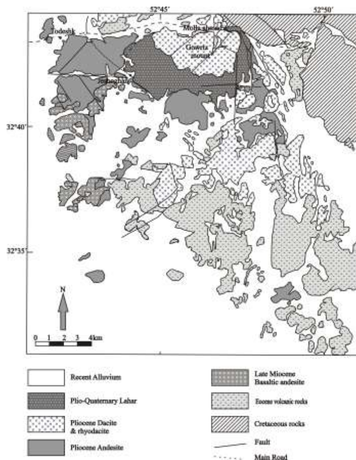
شکل ۳ نقشه‌ی زمین‌شناسی گسترده‌ی مورد بررسی در جنوب شرق اصفهان [۱۳] (اقتباس از نقشه زمین‌شناسی ۱:۱۰۰۰۰۰ کجان، با تغییرات).
