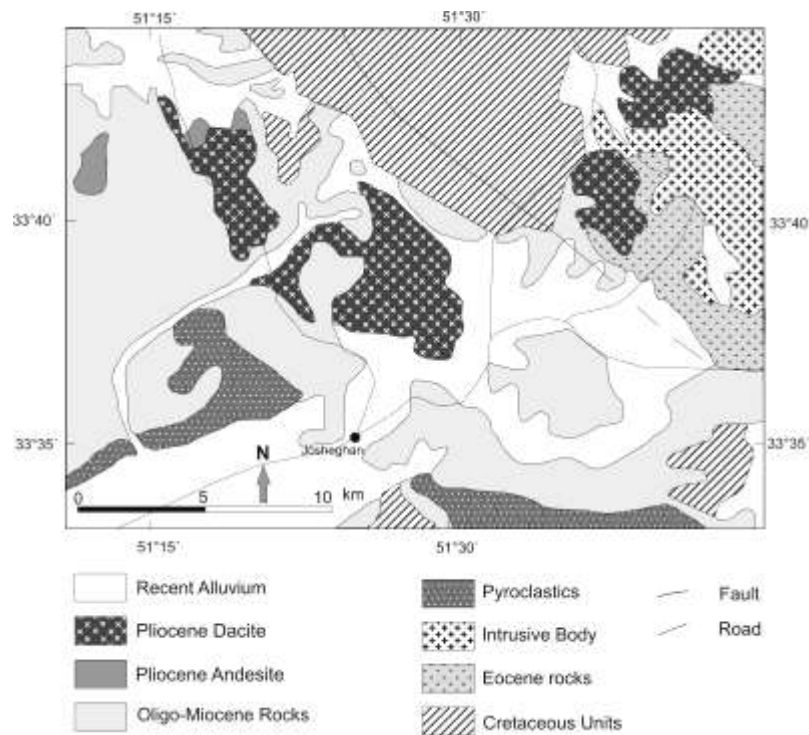
شکل ۲ نقشه‌ی زمین‌شناسی گسترده‌ی مورد بررسی در شمال غربی اصفهان [۱۴] (اقتباس از نقشه زمین‌شناسی ۱:۲۵۰۰۰۰ کاشان، با تغییرات).
