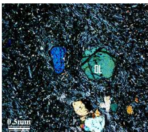
شکل ۳. فنوکریست های الیون کریزولیتی در بازالت XPL.
