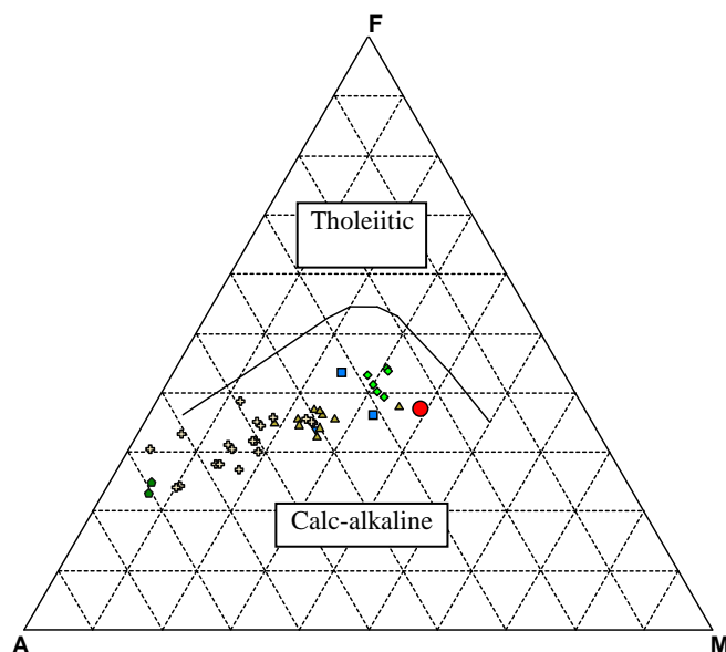
شکل ۲۴ نمودار AFM * ; \text{Na}_2\text{O} + \text{K}_2\text{O} - \text{MgO} - \text{FeO} (Irvine & Baragar, 1971) [۱۳].
