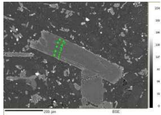
شکل ۱۹. تصویر ریز پردازش بلورهای انستاتیت در سنگ‌های آندزیتی که محل نقاط آنالیز شده روی آن نشان داده شده است.
