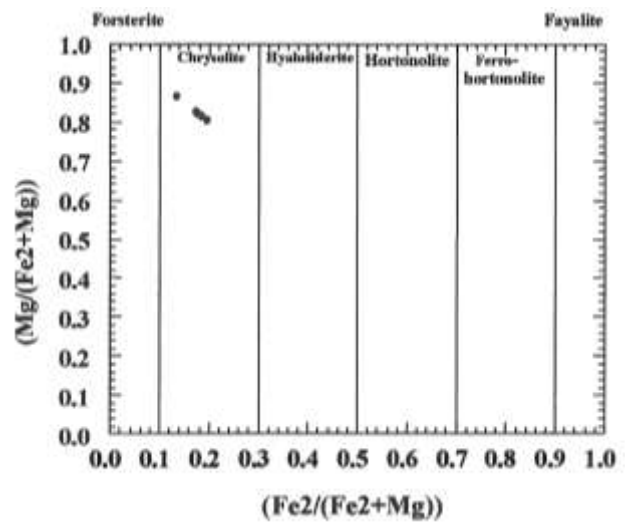
شکل ۷ ترکیب شیمیایی بلورهای الیومین بازالت‌ها و آندزیت‌های بازالتی مورد بررسی.
