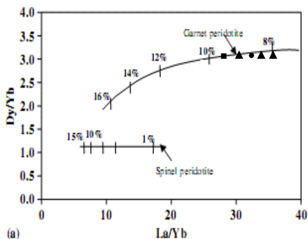
شکل ۱۱ نمودار نسبت Dy/Yb نسبت به La/Yb [۱۸] برای نمونه‌های مورد بررسی خاستگاه گارنت لرزولیت را نشان می‌دهد. علائم مشابه شکل ۴ است.
