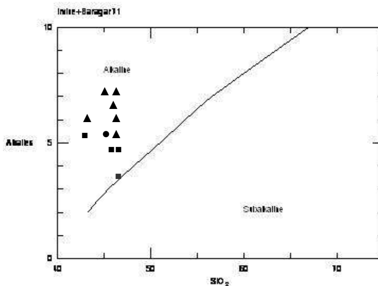
شکل ۵ تعیین سری ماگمایی سنگ‌های بازالتی گستره دریاچه‌ی هامون بر اساس نمودار اروین و باراگار، (۱۹۷۱) [۱۰] علائم مشابه شکل ۴ است.
