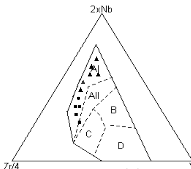
شکل ۸. نمونه‌های مورد بررسی روی نمودار Zr/4-2Nb-Y [۱۴] در گستره‌ی بازالت قلیایی درون صفحات قرار می‌گیرند. علائم مشابه شکل ۴ است. A1: بازالت‌های قلیایی درون صفحات، AII: بازالت‌های قلیایی و تولیت درون صفحات، B: بازالت‌های E-MORB، C: بازالت‌های تولیت درون صفحات و بازالت‌های جزایر قوسی، D: بازالت‌های جزایر قوسی و بازالت‌های N-MORB.
