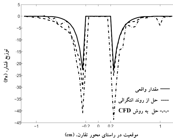
شکل ۱۰- توزیع فشار در محور تقارن مدل جریان کوئنت از محاسبات ریاضی معادله (۳۲) (خط پر) با استفاده از حل انتگرالی حاضر (خط چین) و از روشهای متداول دیفرانسیلی (خط نقطه) وقتی داده های اولیه سرعت با همهمه ترکیب شده اند
