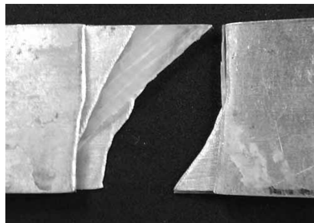
شکل ۷- تصویر شکست نمونه H پس از انجام آزمون کشش.
