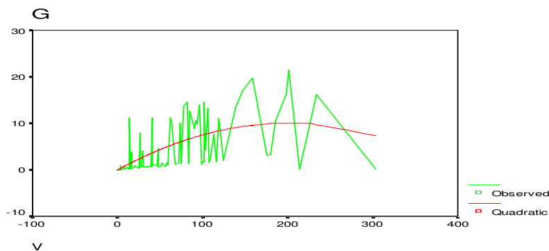
نمودار ۵. تابع رشد بیولوژیک سری ۱۶، حوزه شفارود
