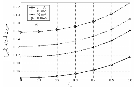
شکل ۱۲ وابستگی مشخصه کوک لیزر به ضریب تلفات C_L به ازای R=R'=0, C_L=0.05, I_{PC}=0
