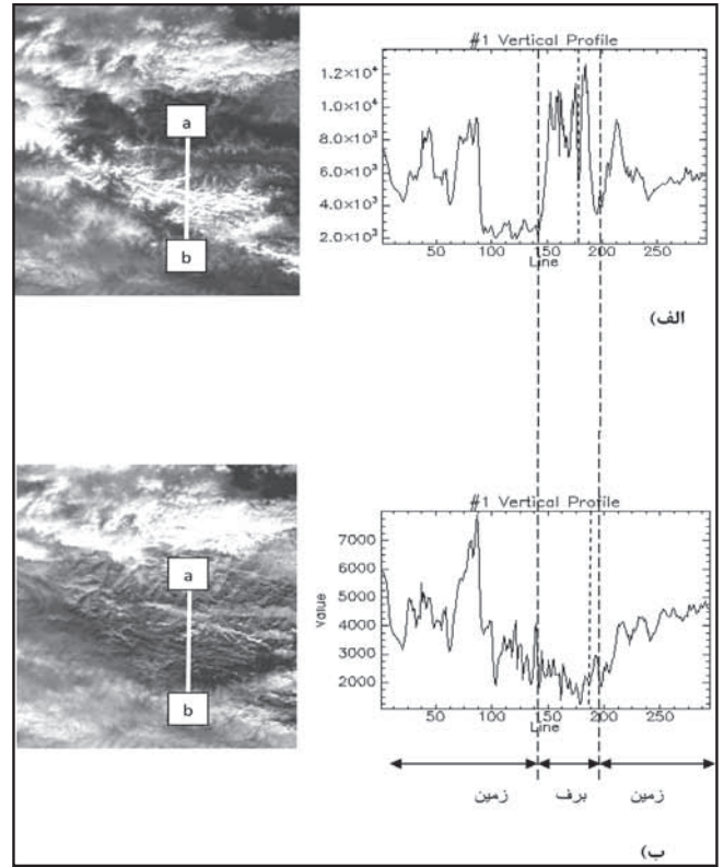
شکل ۴- نیمرخ بازتابی در تصویر تاریخ ۲۰۰۲/۱/۶، الف) باند مرئی ب) باند مادون قرمز میانی
