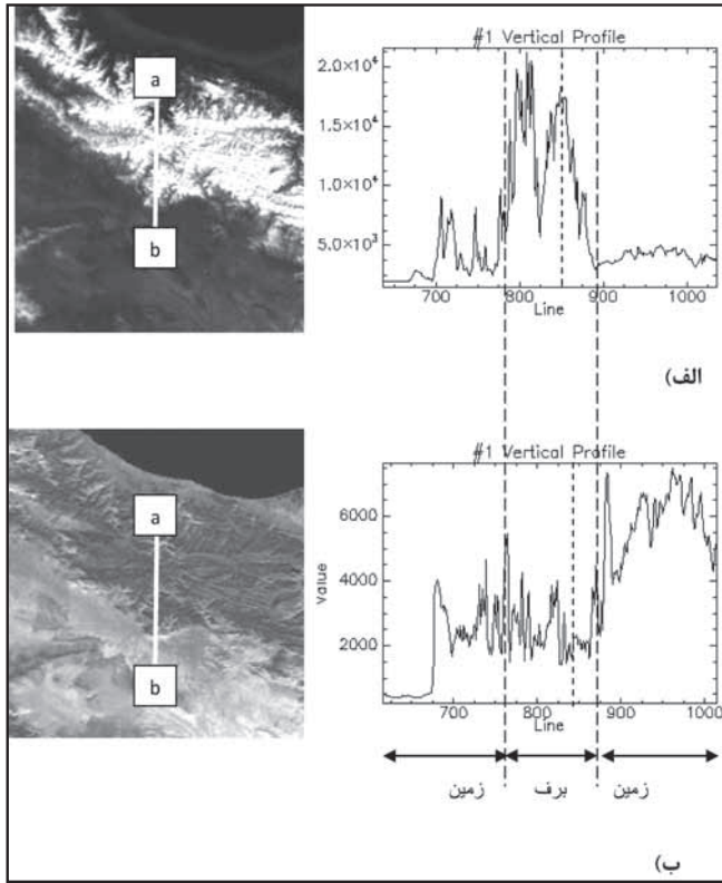
شکل ۳- نیمرخ بازتابی در تصویر تاریخ ۲۰۰۲/۲/۲، الف) باند مرئی ب) باند مادون قرمز میانی
