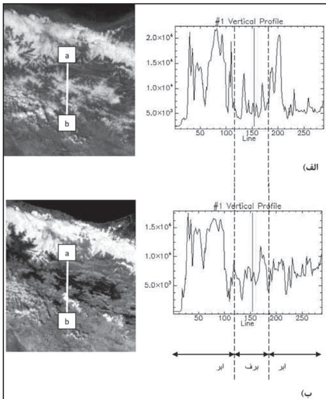
شکل ۵- نیمرخ بازتابی در تصویر تاریخ ۲۰۰۲/۴/۳۰، الف) باند مرئی ب) باند مادون قرمز میانی
