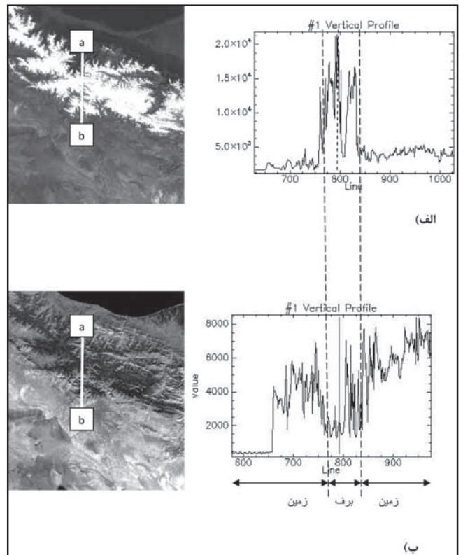
شکل ۶- نیمرخ بازتابی در تصویر تاریخ ۲۰۰۲/۳/۲، الف) باند مرئی ب) باند مادون قرمز میانی
