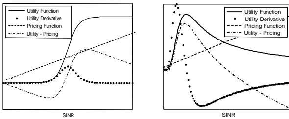
شکل ۳: نمونه‌ای از توابع بهره دسته سوم و چهارم به ترتیب از سمت چپ، همراه با مشتق تابع، تابع هزینه و تابع بهره.
