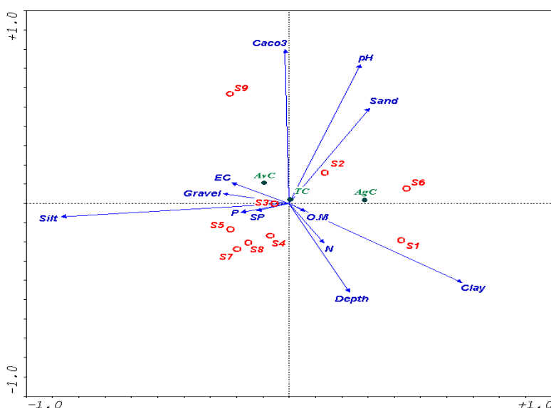
شکل ۱* - نمودار سه پلاتی گونه-عوامل خاک- مکان حاصل از آنالیز رج‌بندی به روش CCA
