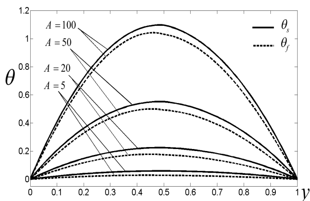
شکل ۳ توزیع دمای فاز سیال و جامد در ماده متخلخل در ضرایب انتقال حرارت مختلف به ازای k=0.1 ، \epsilon_1=0.4 و \epsilon_2=0.8
