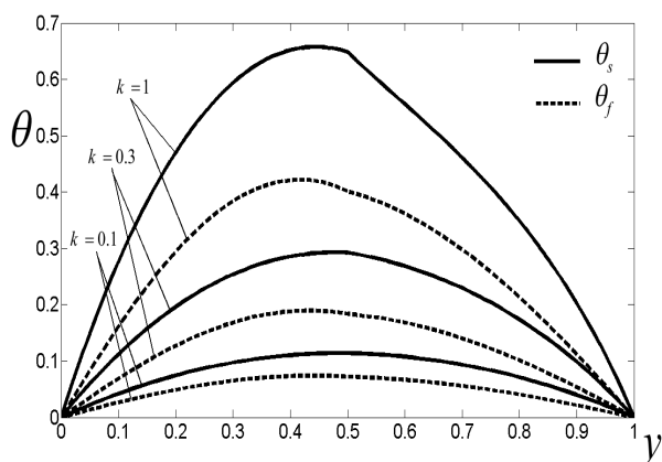
شکل ۲ توزیع دمای بدون بعد فازهای سیال و جامد در ماده متخلخل در نسبت‌های ضریب هدایت حرارتی مختلف به ازای A=10 ، \epsilon_1=0.4 و \epsilon_2=0.8
