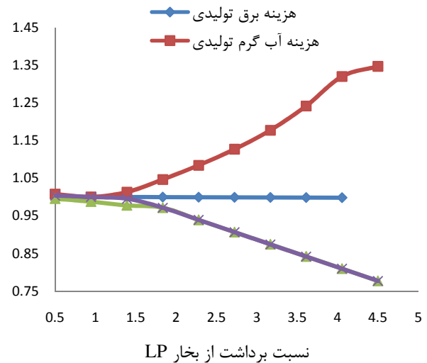
شکل ۴ تاثیر دبی بخار LP برداشتی بر هزینه تولید توان، هزینه تولید آب، راندمان انرژژی و انرژژی سیکل
