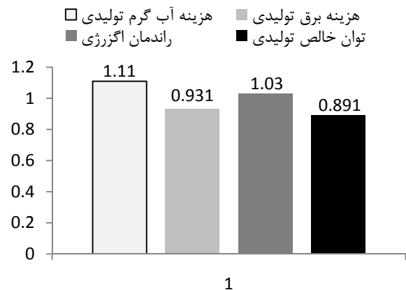
شکل ۹ نسبت هزینه تولیدی محصولات، دبی آب گرم تولیدی و راندمان انرژی حالت بهینه به حالت پایه
