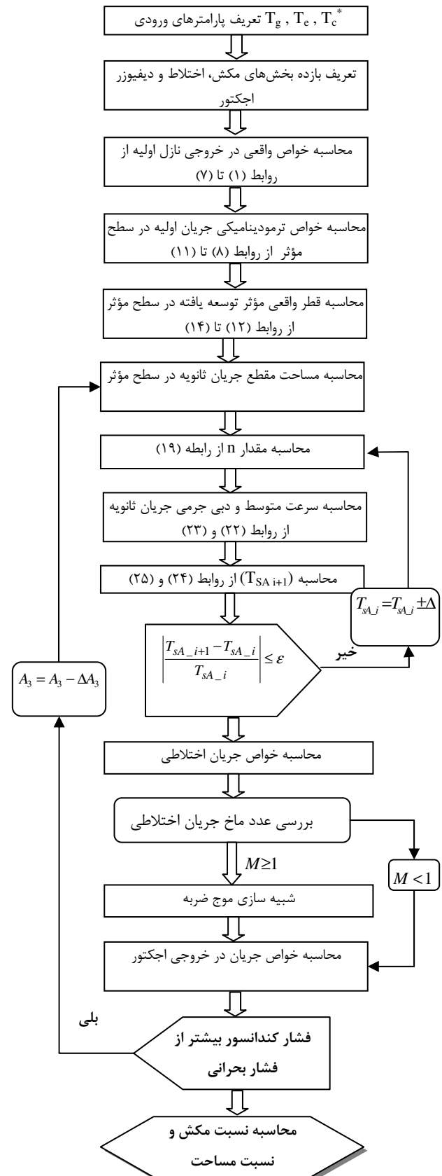
شکل ۷ نمودار گردش مدل ترمودینامیکی
