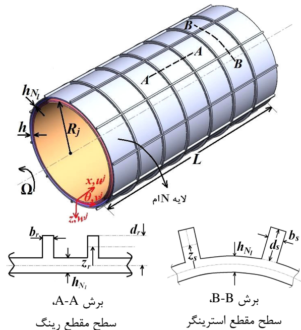
شکل ۱ هندسه و نمادگذاری پوسته استوانه‌ای تقویت‌شده
