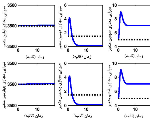
شکل ۷ نمایش پارامترهای میراکننده مجازی به‌روزشده برای صفحات خورشیدی برای کنترل تطبیقی ترکیبی خنثی‌کننده (پارامتر تخمین زده شده — N.m/sec واقعی - - - N.m/sec)
